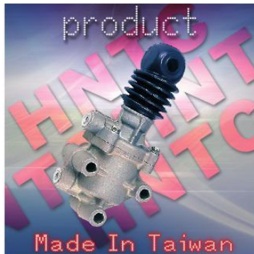
CYLINDER, GEARSHIFT 高低檔控制缸總成 行程25mm M12-3S10 FV415 ME652800 661-00518 CYLINDER, GEARSHIFT 高低檔控制缸總成 行程30mm FP517 FV515 M120 ME671397
