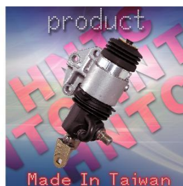
SERVO, GEARSHIFT 變速補助缸 RH 十字型 LFS*98 GH FG FM2P 33510-1270 33510-1450 654-04505 33510-1431 R/KIT:33590-1210
