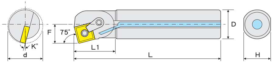
d = 最小車徑 d = Min. Bore Dia. / 右車刀桿圖示 Right-Hand Shown
